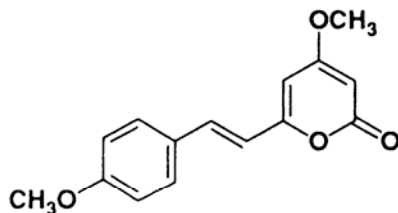
Yangonin
